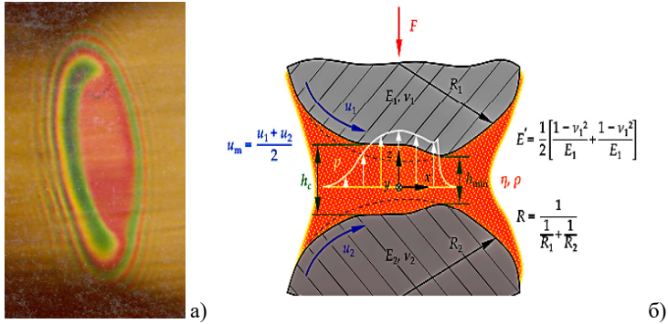
Рис. 1. Розподіл товщини мастильного шару (а) та схематичне зображення лінійного ЕГД-контакту із відповідними змінними для чисельних розрахунків (б).
